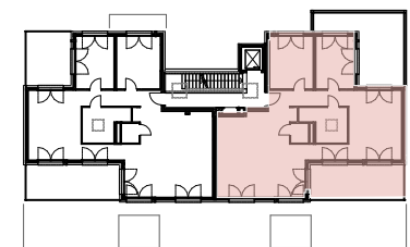
Übersicht 2. Dachgeschoss
